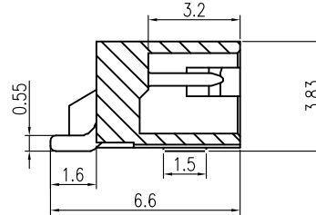
截面 A-A
